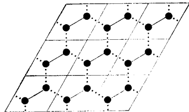
Фиг. 4.17. Сеть «пчелиных сот», изображенная таким образом, чтобы подчеркнуть, что она представляет собой решетку Бравэ с двухточечным базисом.
