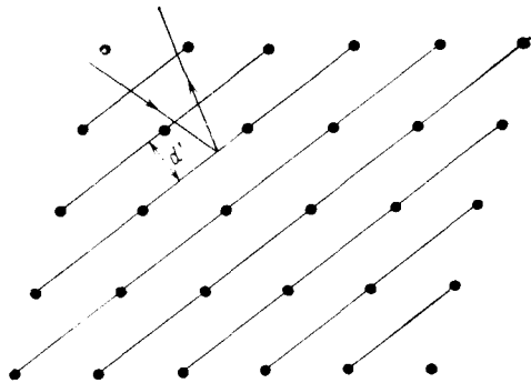
Фиг. 6.3. Иное разбиение на атомные плоскости части решетки Бравэ, показанной на фиг. 6.1.
