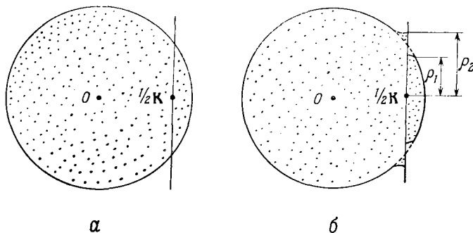
Фиг. 9.6. а — сфера свободных электронов, пересекающая брэгговскую плоскость, удаленную на 1/2\mathbf{K} от начальной точки ( U_{\mathbf{k}} = 0 ); б — искажение сферы свободных электронов вблизи брэгговской плоскости при U_{\mathbf{k}} \neq 0 . Поверхность постоянной энергии пересекает плоскость по двум окружностям, радиусы которых вычисляются в задаче 1.
