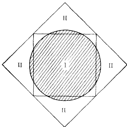
Фиг. 12.3. Двумерный пример, поясняющий, почему двухвалентное твердое тело может быть проводником.
