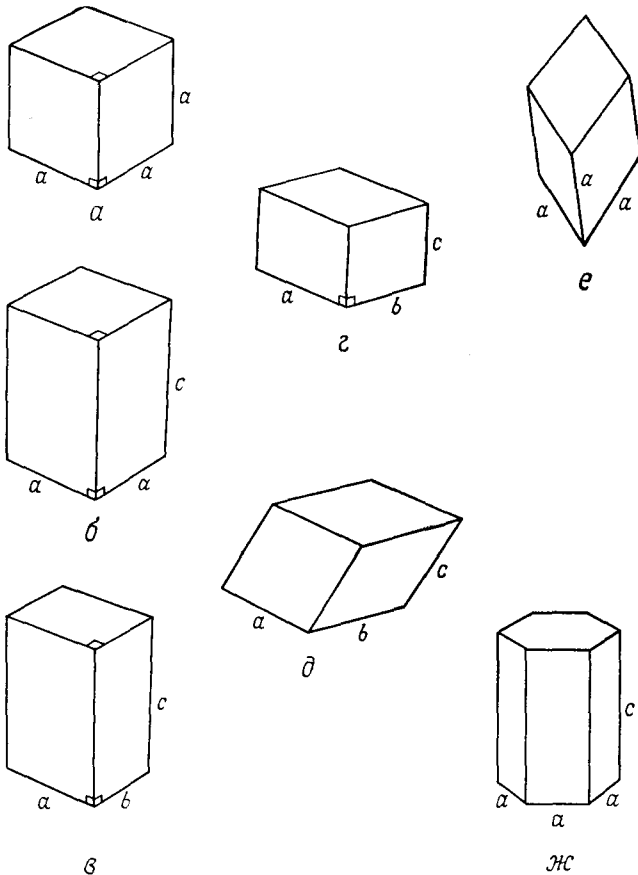
Фиг. 7.3. Объекты с симметриями точечных групп решеток Бравэ, принадлежащих семи кристаллическим системам: кубической ( а ), тетрагональной ( б ), ромбической ( в ), моноклинной ( г ), триклинной ( д ), тригональной ( е ), гексагональной ( ж ).
