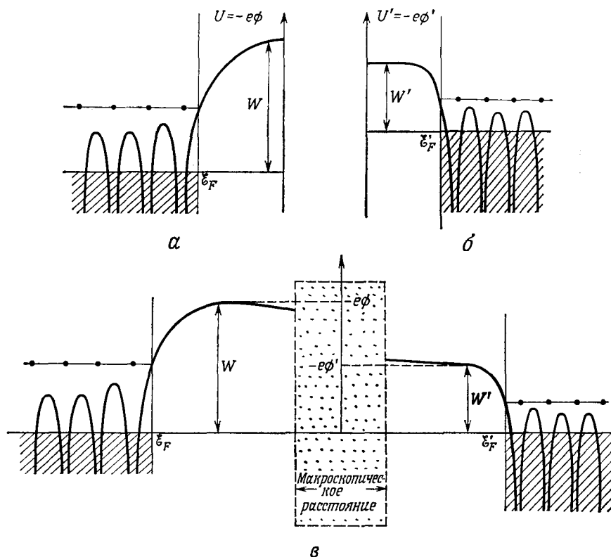
Фиг. 18.4. \alpha — кристаллический потенциал U [или электростатический потенциал \phi = U/(-e) ] для металла с работой выхода W и энергией Ферми \epsilon_F . (Эта фигура совпадает с фиг. 18.2, б.)
