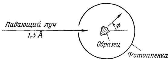
Фиг. 6.13. Схематическое изображение камеры Дебая — Шеррера. Дифракционные максимумы регистрируются на полоске фотопленки.
