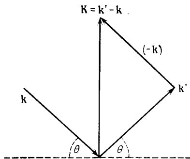
Фиг. 6.6. Волновой вектор k падающего луча, волновой вектор k' отраженного луча и вектор их разности K = k' - k , удовлетворяющий условию Лауэ.
